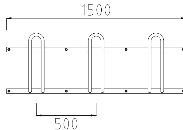
整組平面圖
