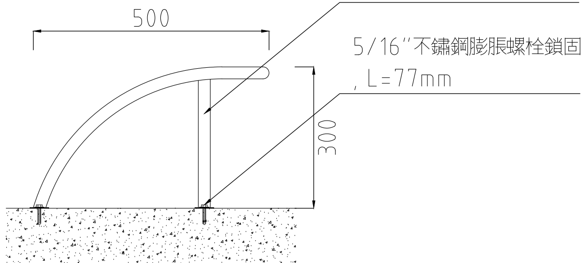
立面圖
