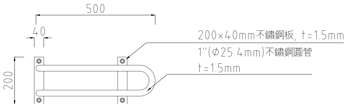
平面圖
