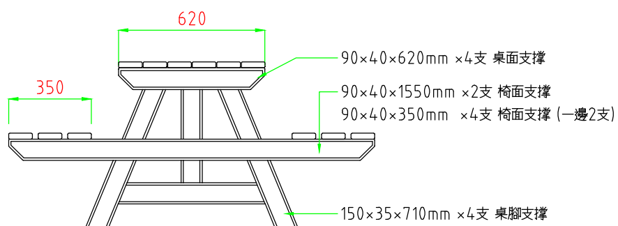
立面圖
