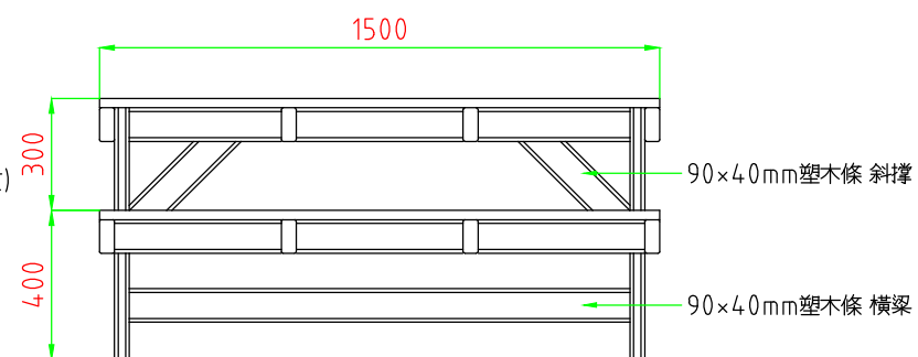
側立面圖
