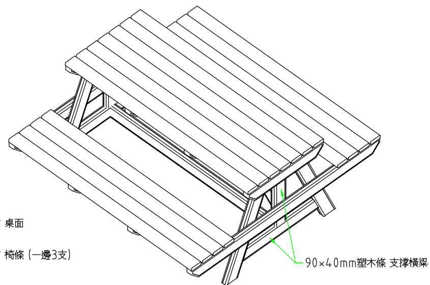
正等軸圖
