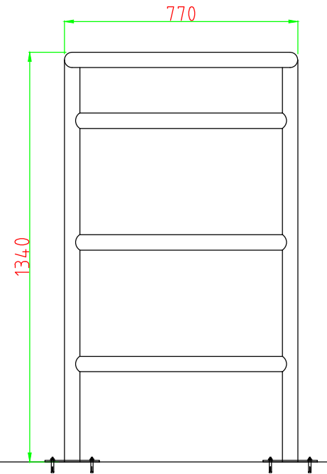
側視圖
