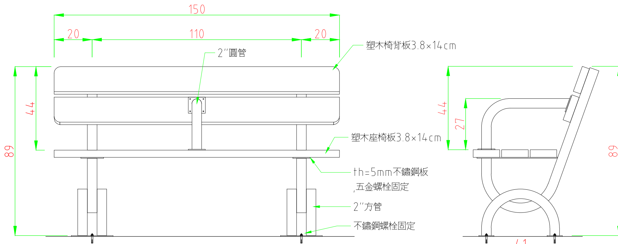
正視圖
