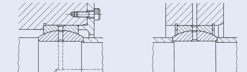
图10 安装例
