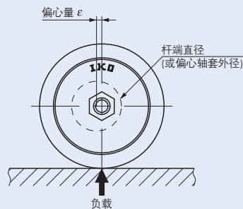
图5 调整偏心杆端凸轮从动轴承及附带偏心轴套的凸轮从动轴承的基准位置
