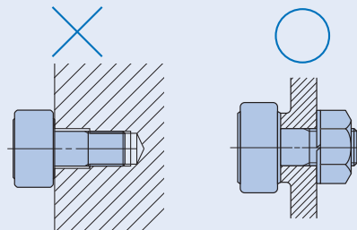
图4 安装方法
