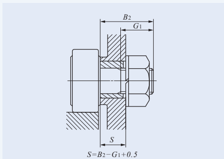
图8 附带偏心轴套的安装孔的长度
