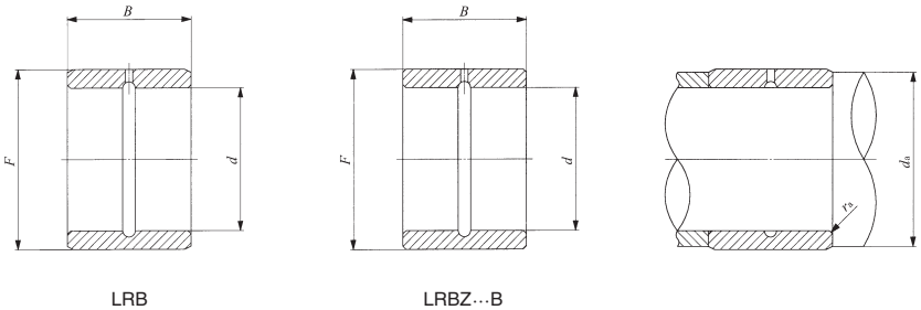
搭配的轴承
