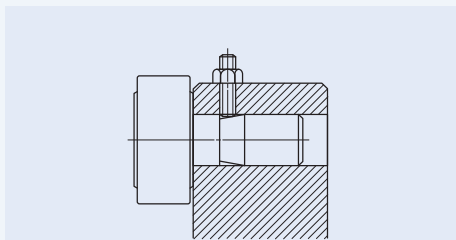
图9 简易安装用凸轮从动轴承的安装例
