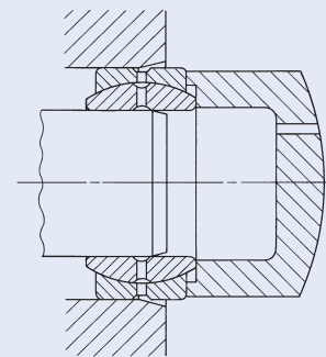
同时安装内圈和外圈时
