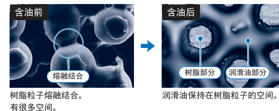
IKO C-Lube自润滑凸轮从动轴承
