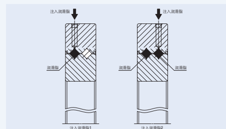
图6 加油方法
