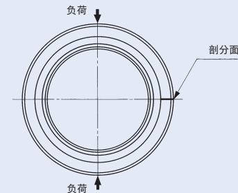
图8 外圈的剖面与负荷方向
