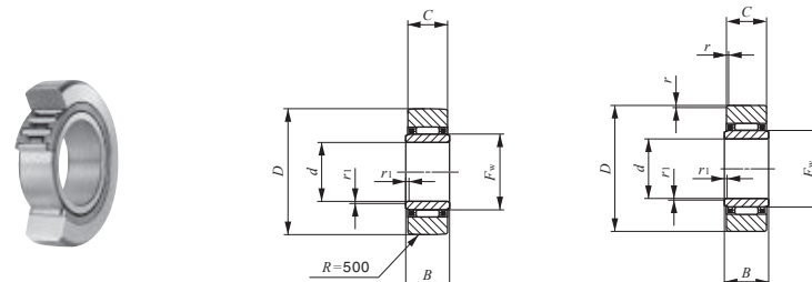
轴径6-50mm
