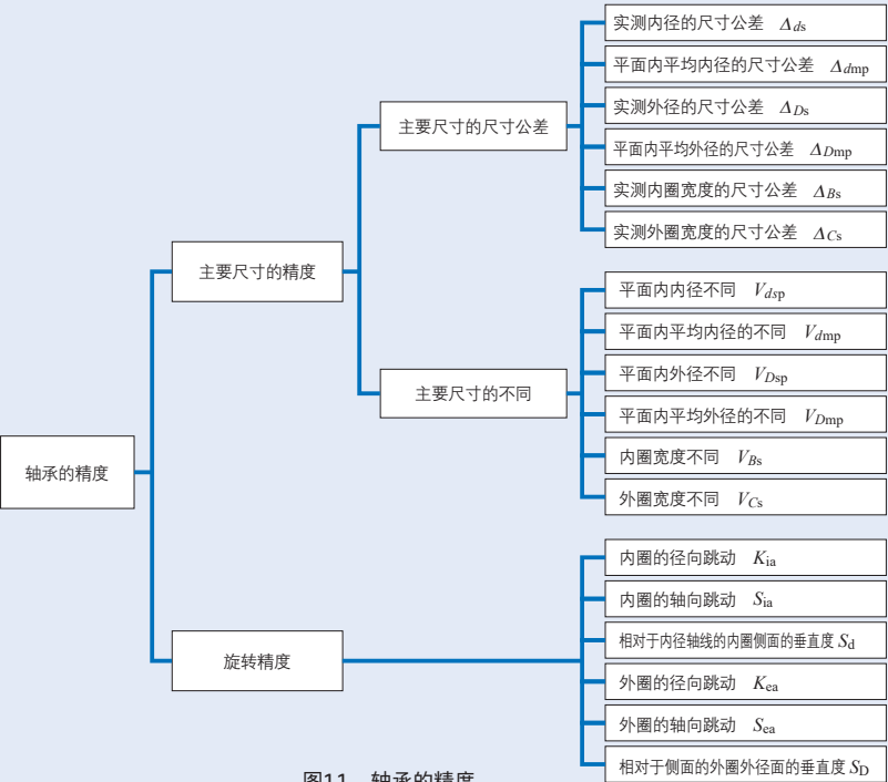
图11 轴承的精度
