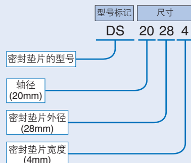
公称型号的排列例
