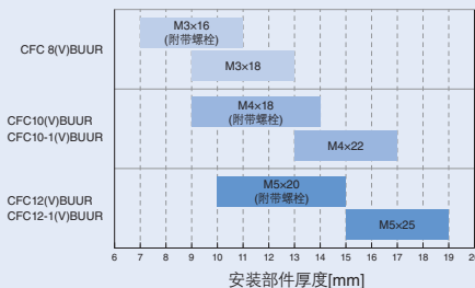
图7 安装用内六角螺栓的选择
