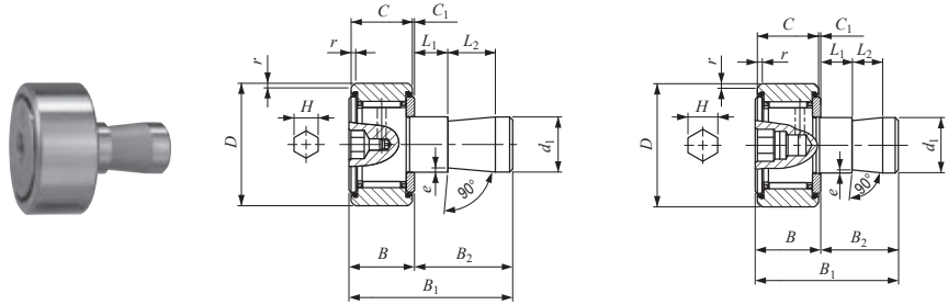
杆端直径6-20mm
