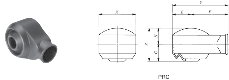
L 型杆端关节轴承用防尘罩
