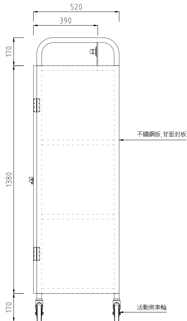
側立面圖
