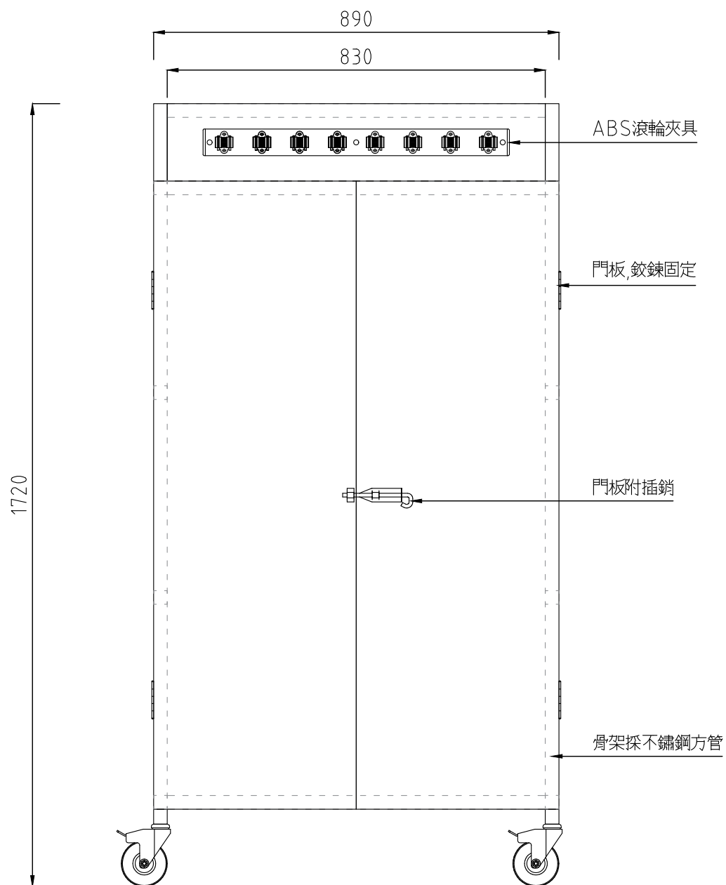
立面圖
