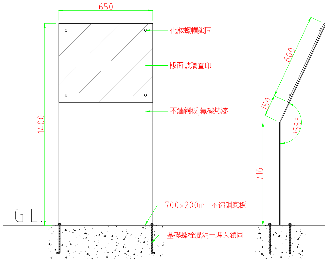
立面圖
