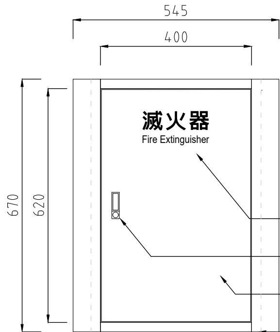
立面圖
