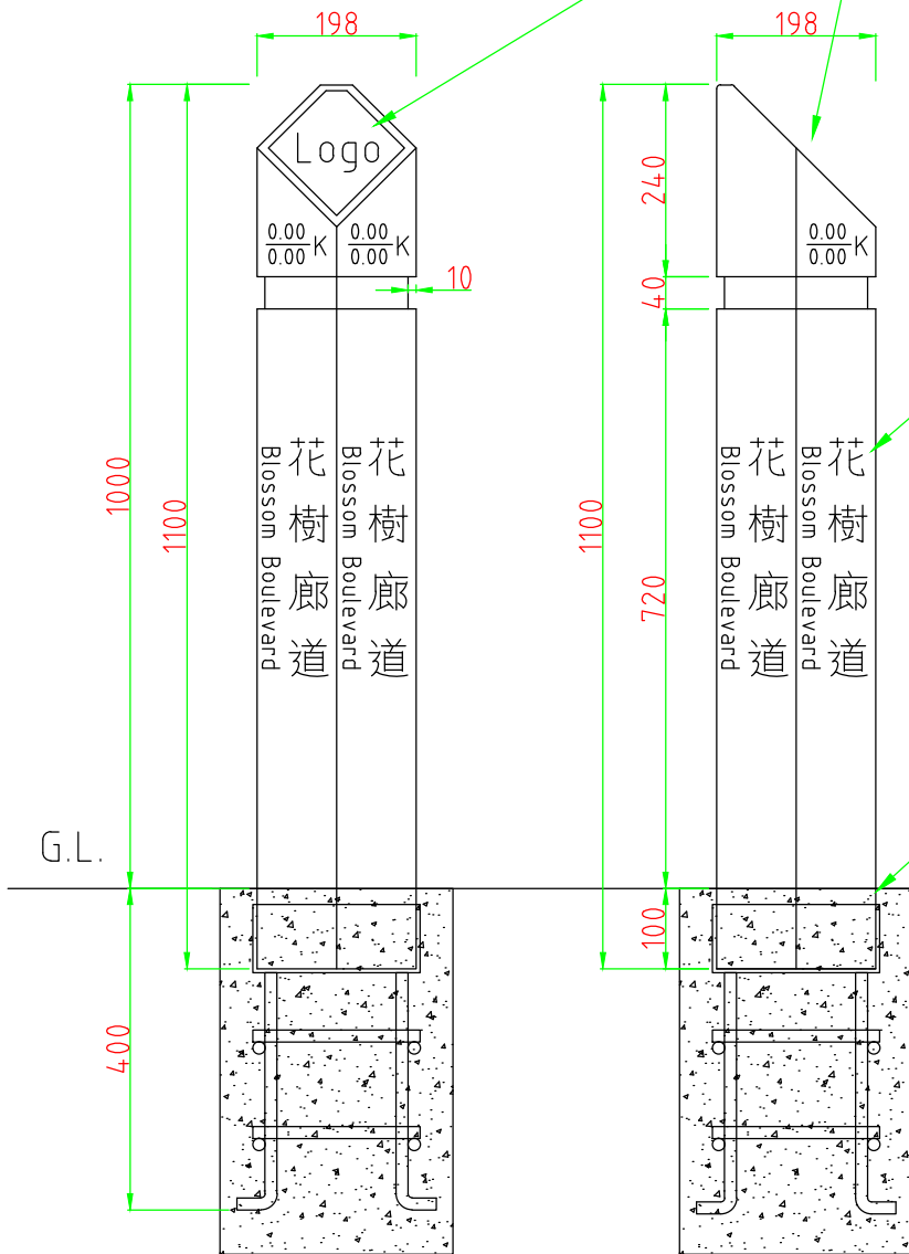
正立面圖
