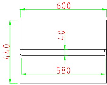
平面圖
