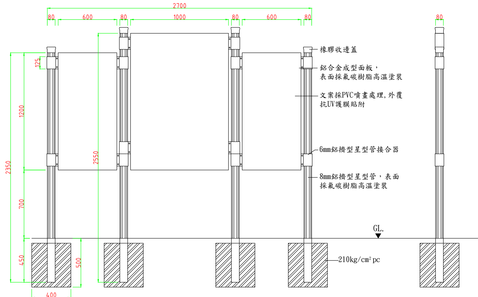
正立面圖
