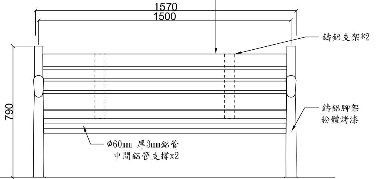
立面圖
