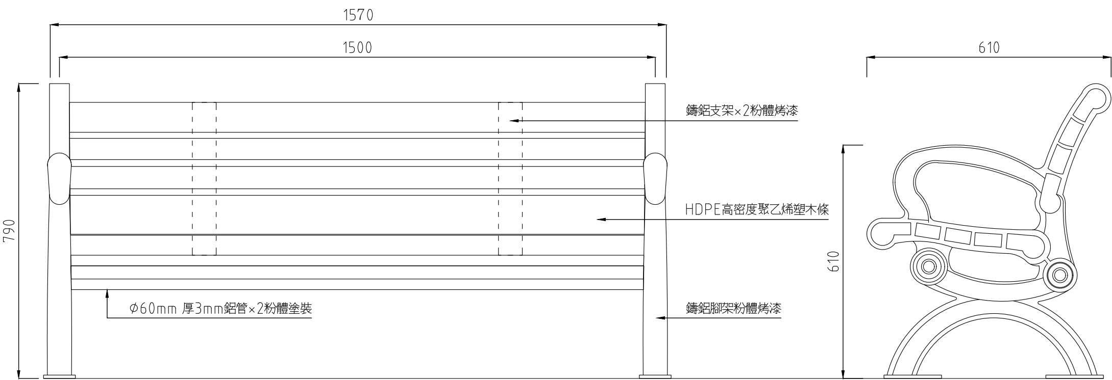
立面圖
