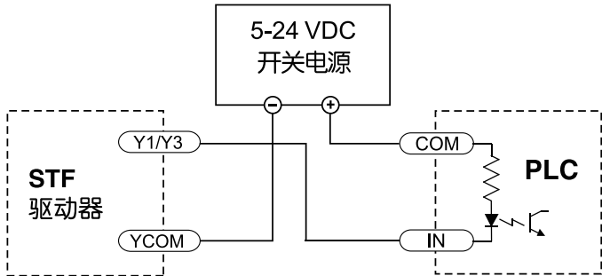
将输出Y1/Y3接成sinking型输出, 与PLC的输入相连
