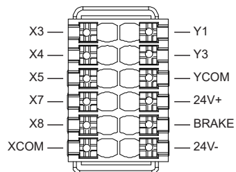
I/O连接器
