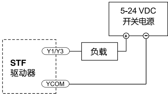
将输出Y1/Y3接成sinking型输出
