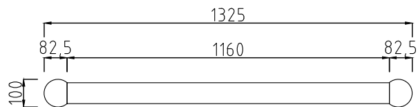
平面圖
