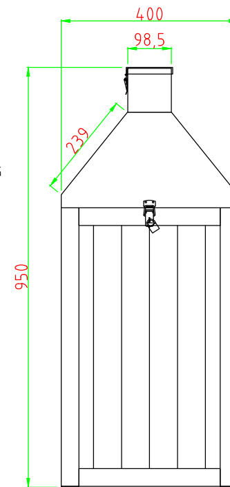
側視圖
