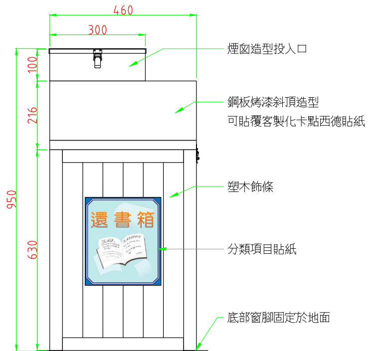
正視圖
