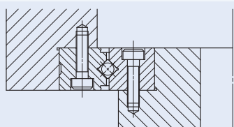
图4 附带安装孔的高刚性交叉滚子轴承直接安装于轴承座之安装例
