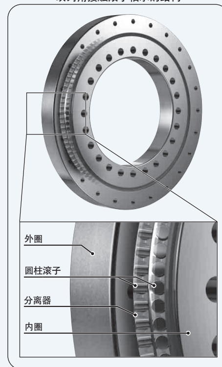
双列角接触滚子轴承的结构
