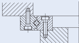
图3 附带安装孔的高刚性交叉滚子轴承直接安装于对方安装面之安装例
