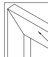
轉角接合詳圖
