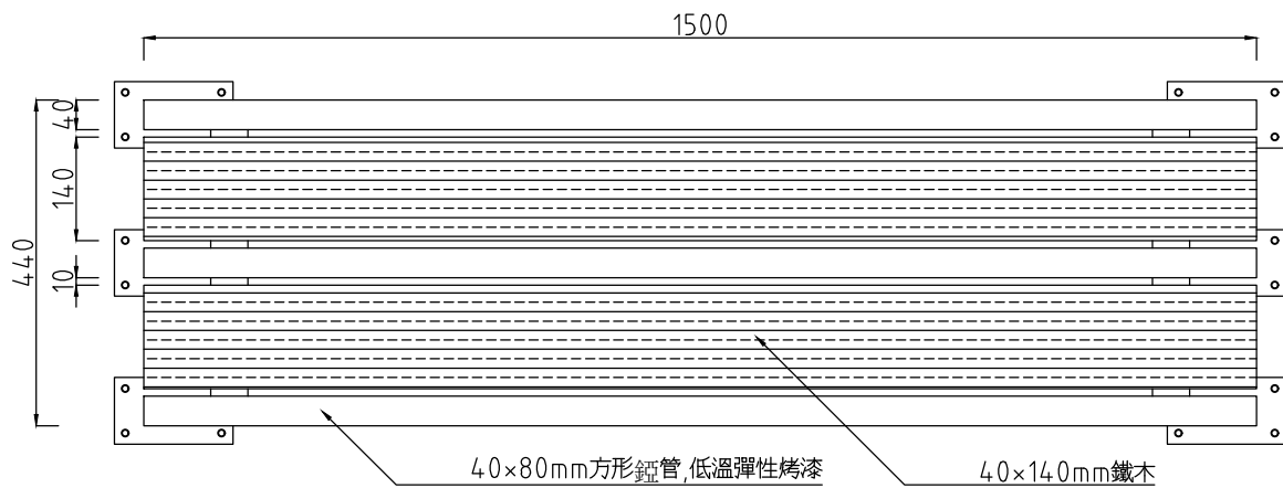
平面圖
