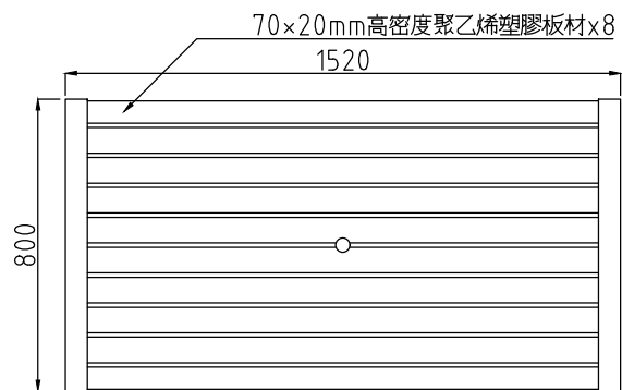
桌子平面圖
