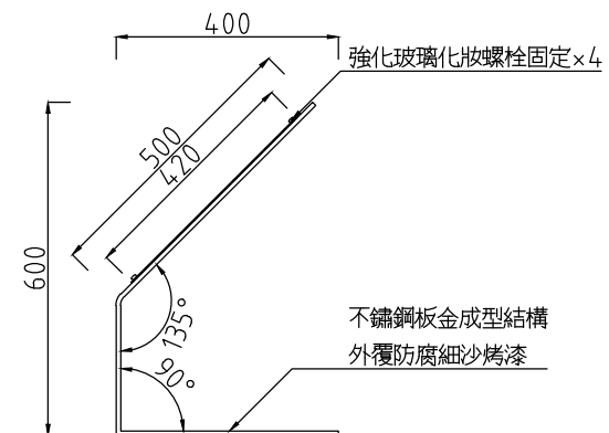
側立面圖
