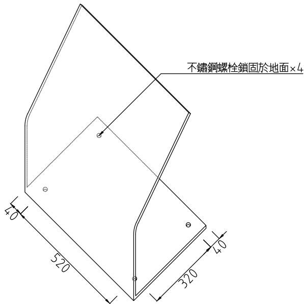
螺栓孔位示意圖
