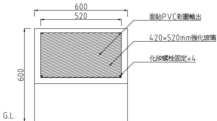
立面圖
