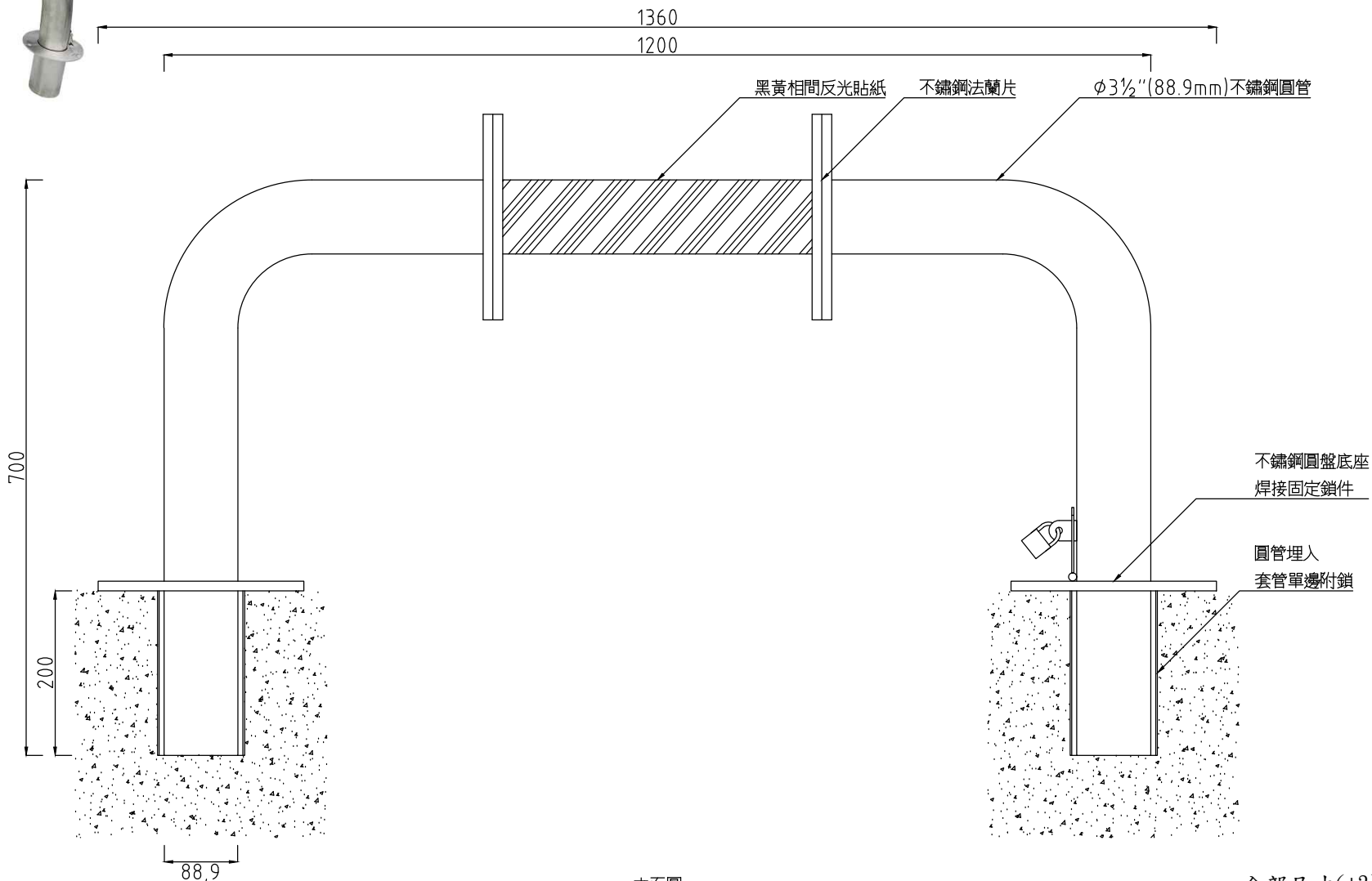
立面圖
