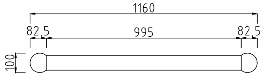
平面圖
