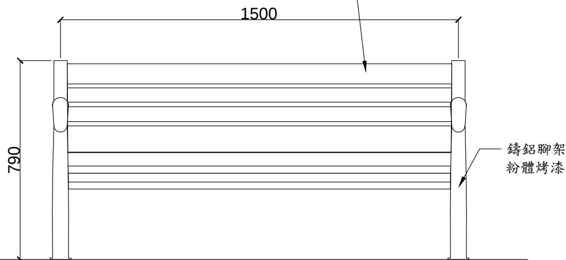
立面圖
