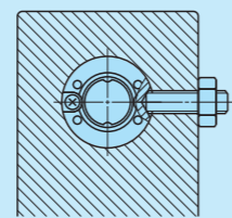
大小尺寸为2、3、4的外筒止转
