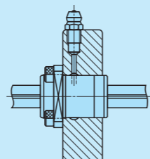
法兰型安装示例
