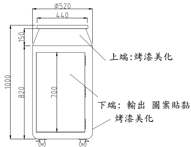
背視圖
