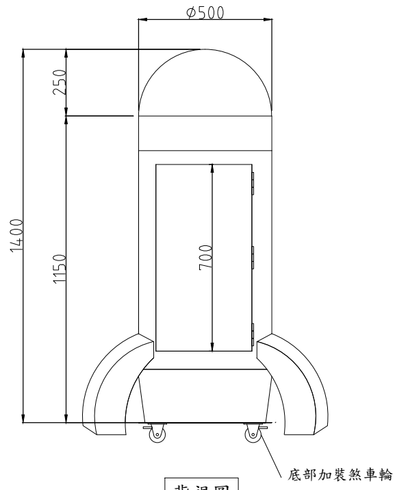
背視圖
