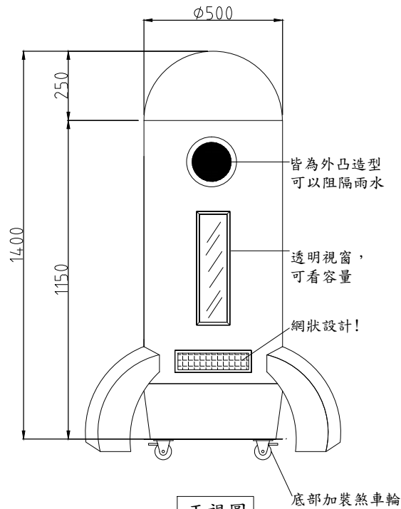
正視圖
