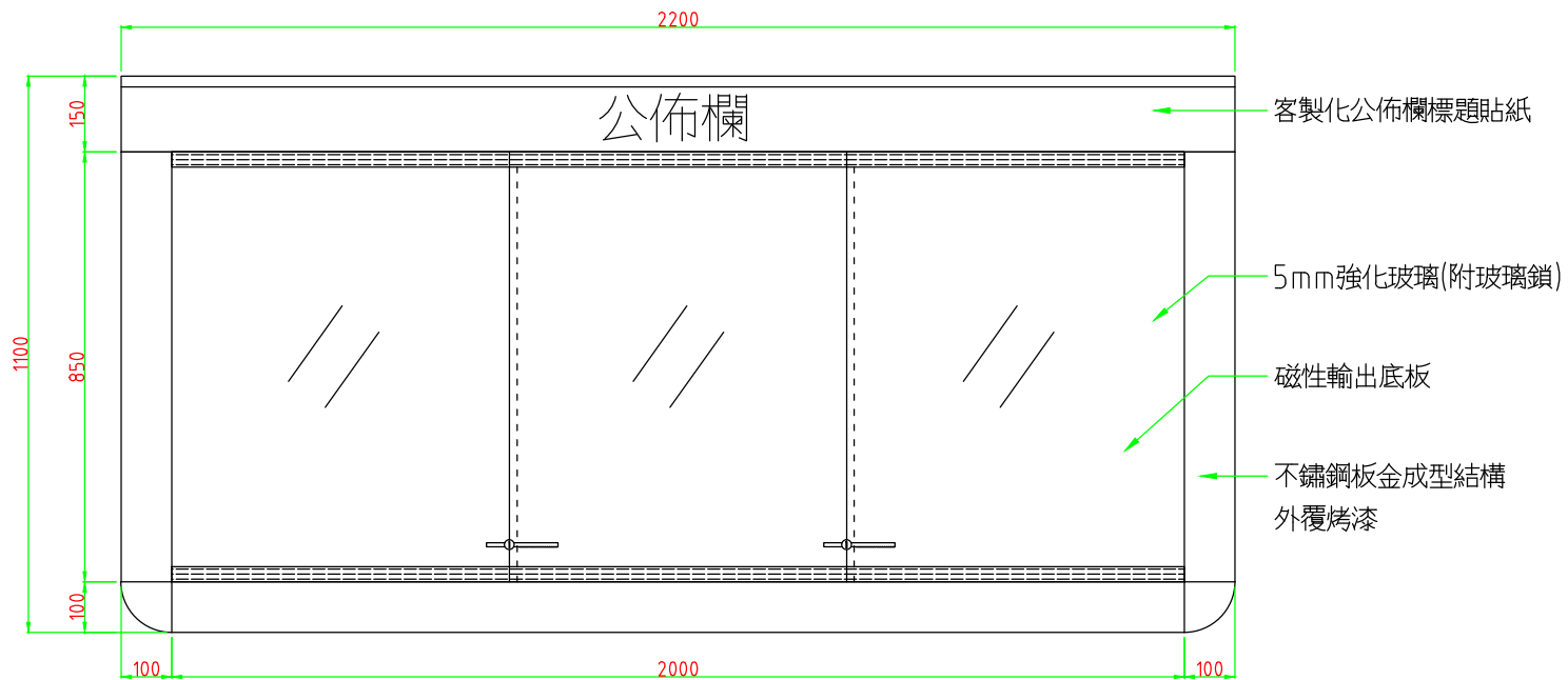
正視圖
