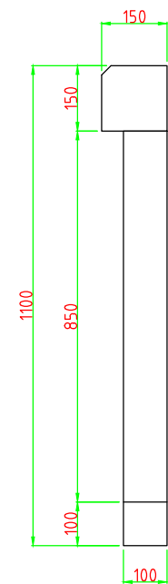
側視圖
