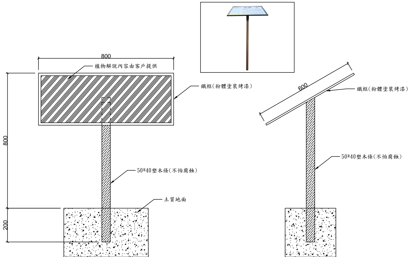
立面圖
