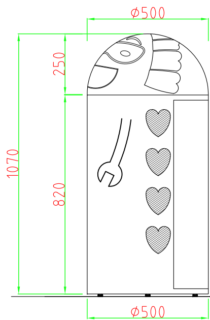
側視圖
