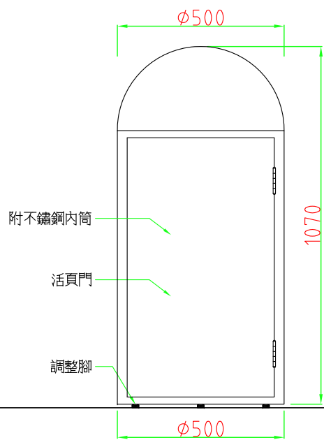
後視圖
