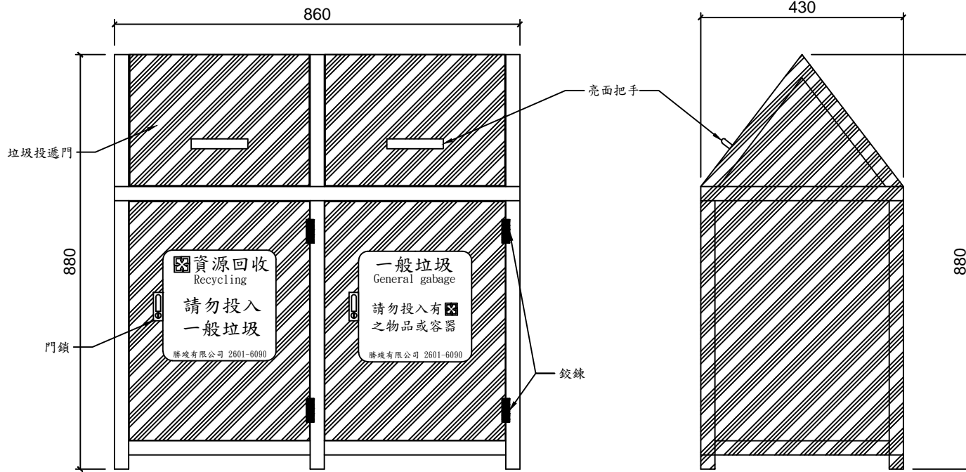
立面圖
