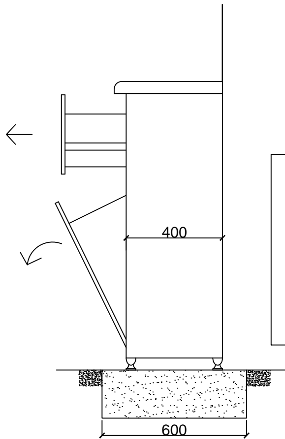
側視圖
