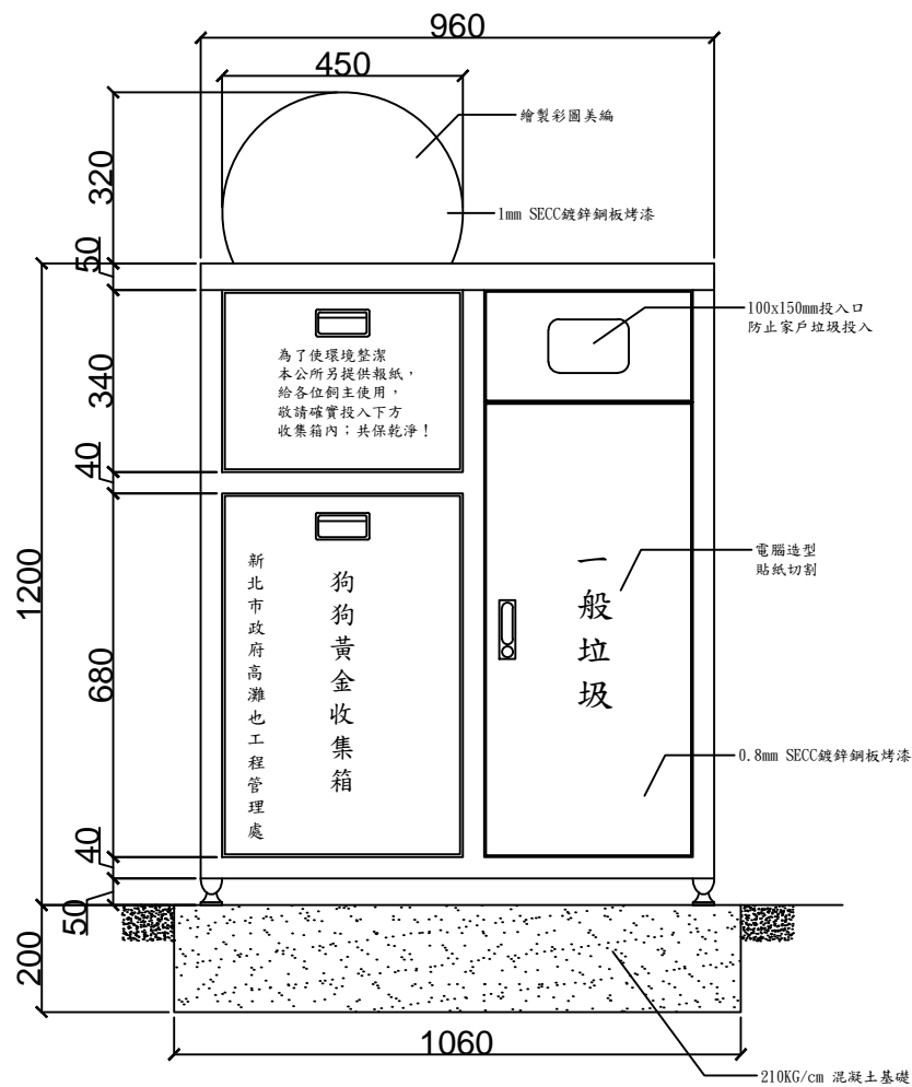
立面圖
