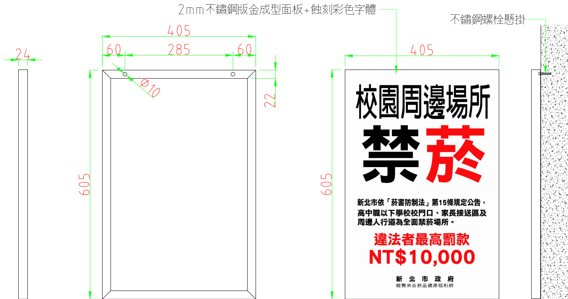
側立面圖
