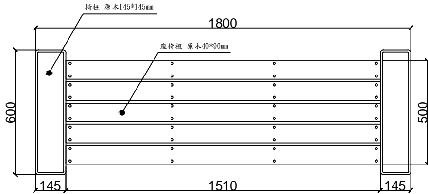
平面圖
