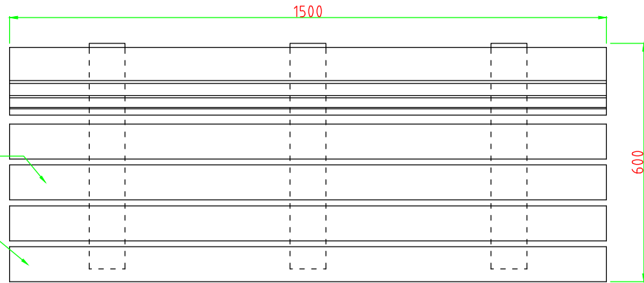
上視圖
