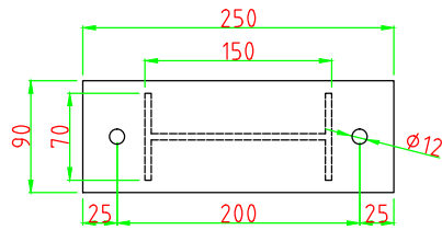
250×90mm, t=9mm 不鏽鋼底板
