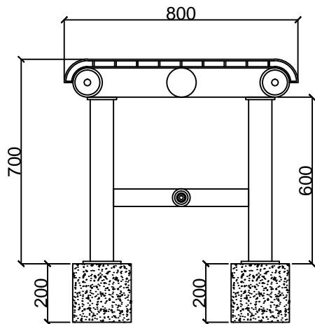
桌子側面圖
