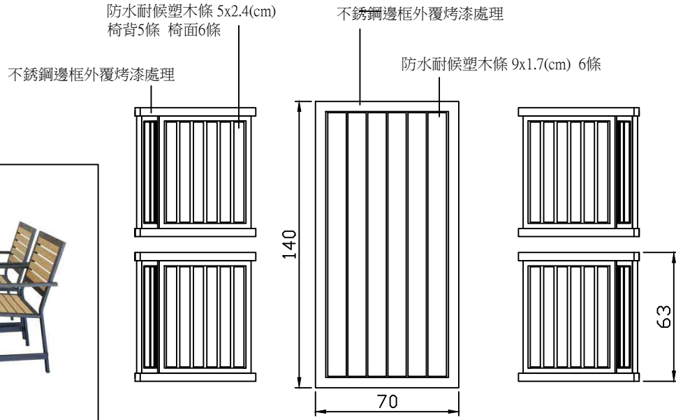
上視平面圖
