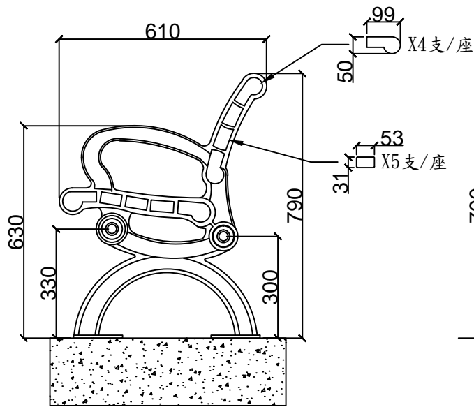
側立面圖
