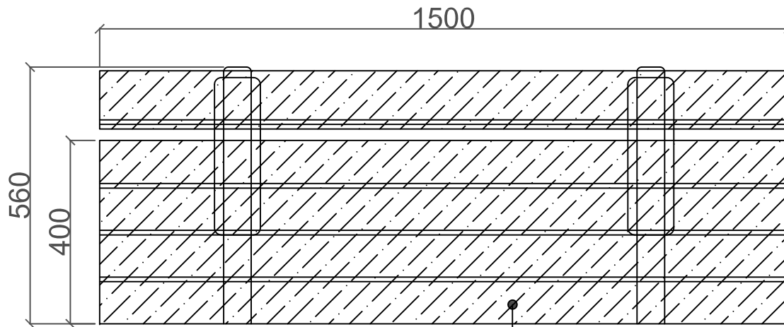
平面圖
