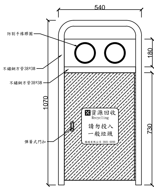
正立面圖
