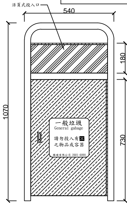
正立面圖
