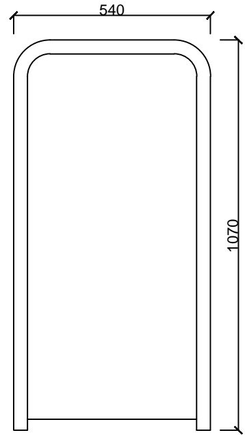
背立面圖
