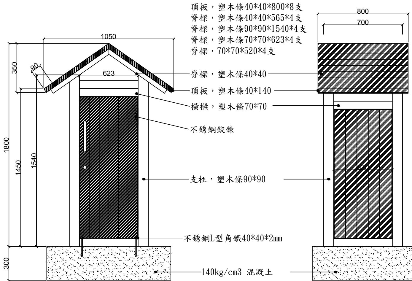
立面圖
