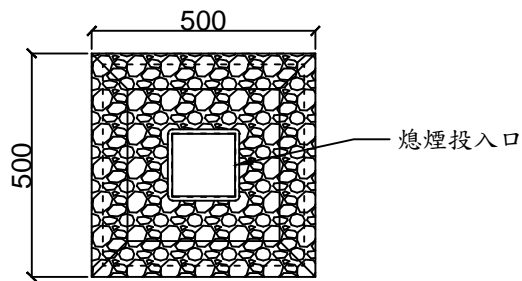
上視平面圖
