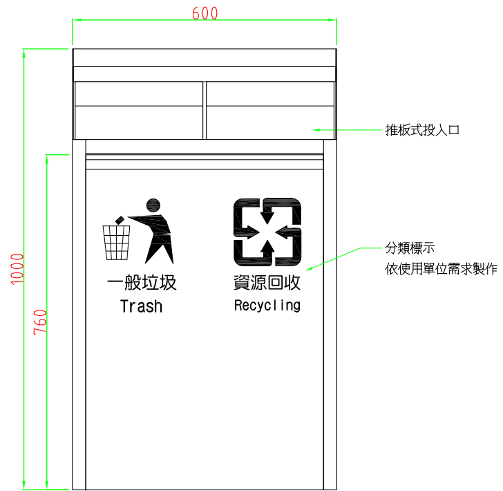
正視圖
