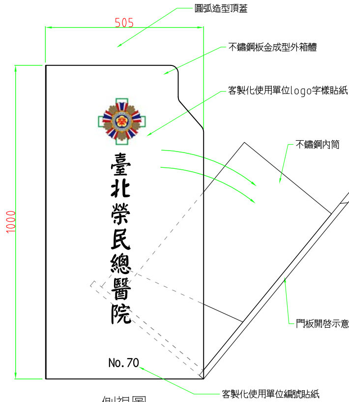
側視圖
