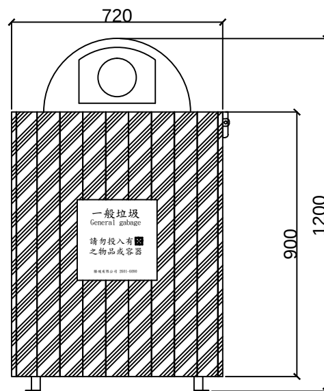
立面圖
