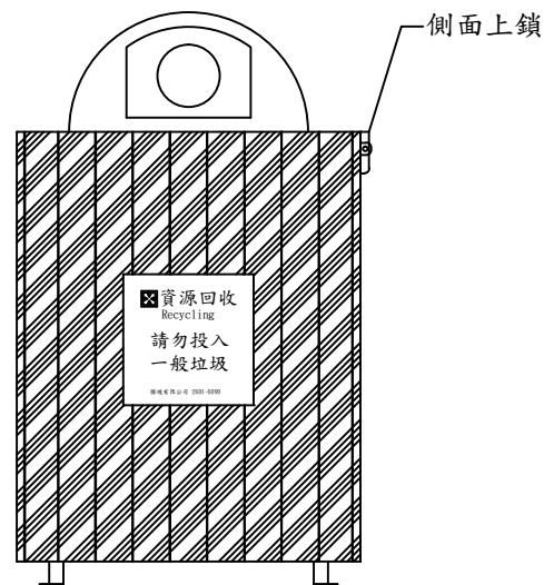
立面圖
