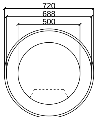
平面圖
