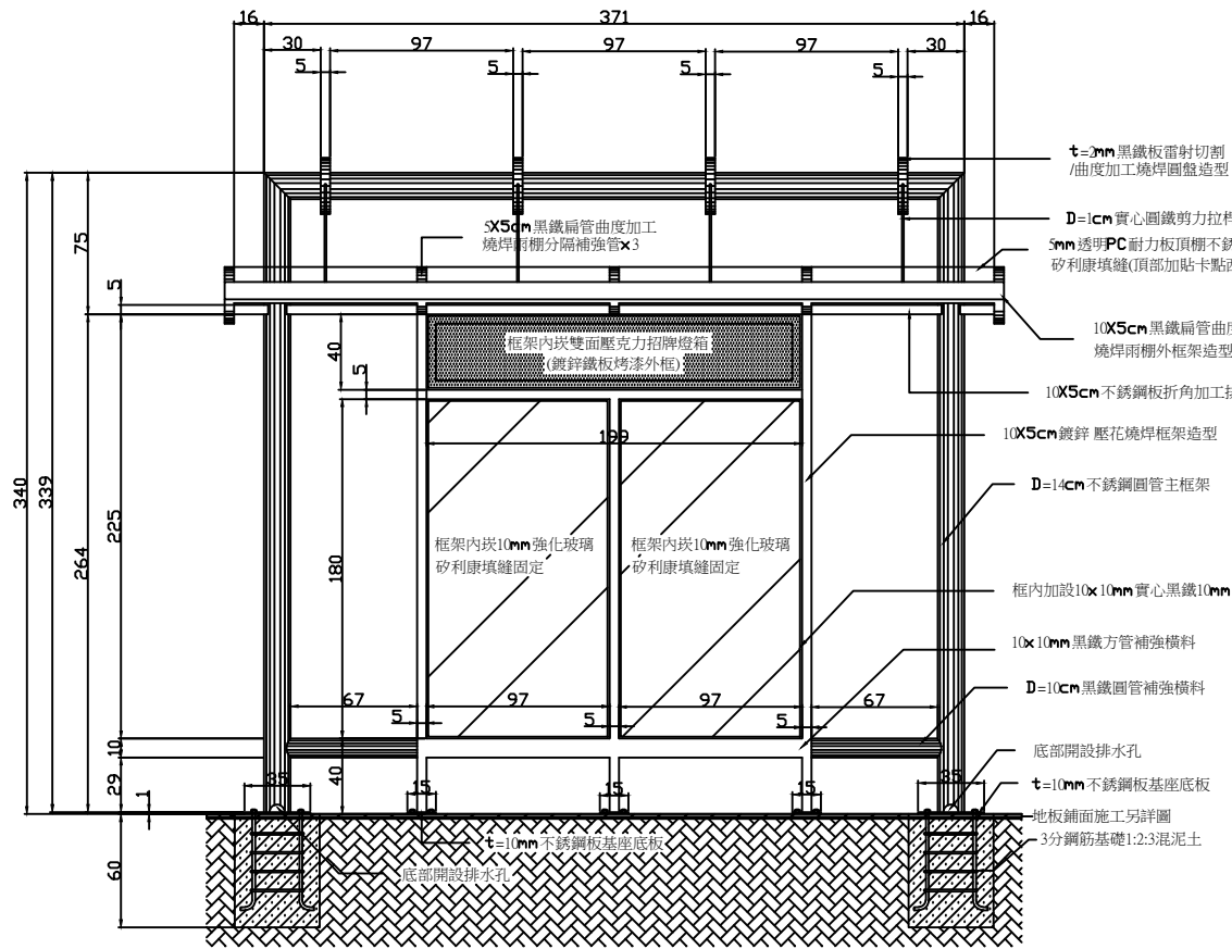
背立面圖
