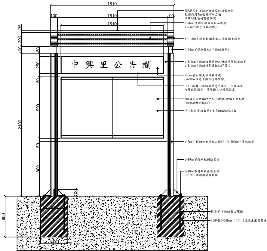
正立面圖
