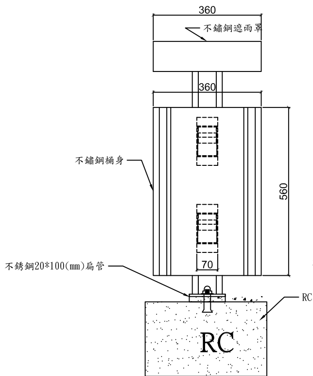
正立面圖
