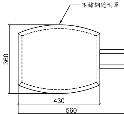
平面圖
