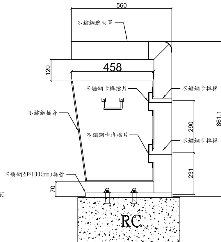
側立面圖
