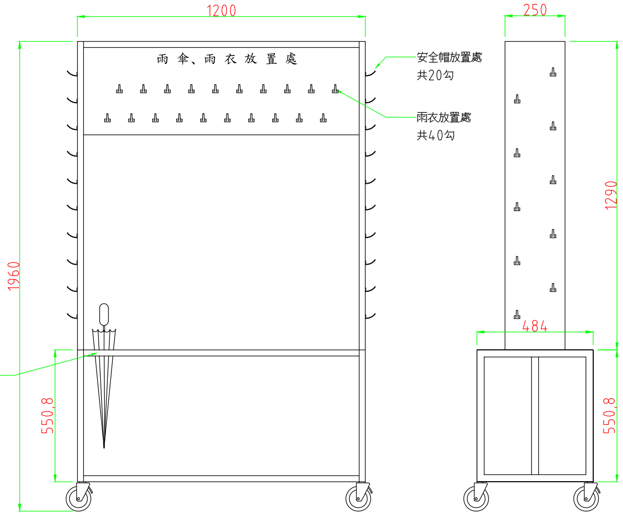
正視圖
