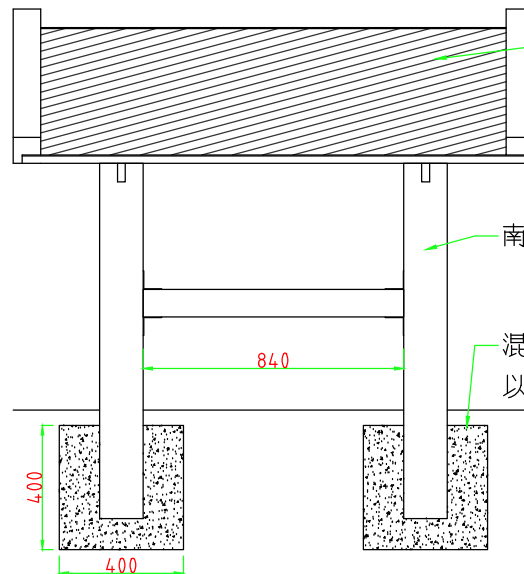
立面圖
