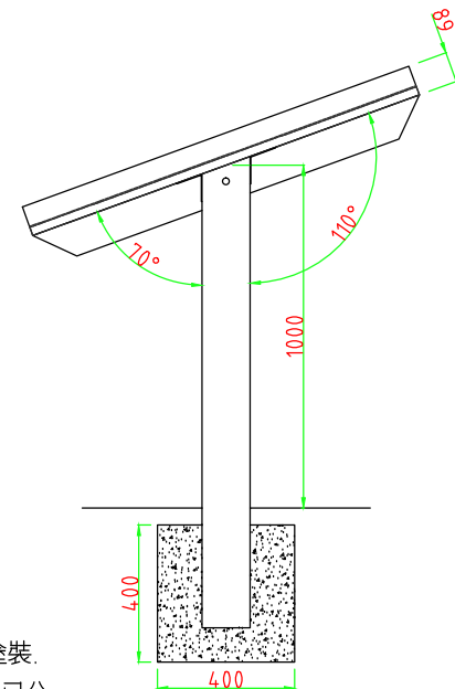
側立面圖
