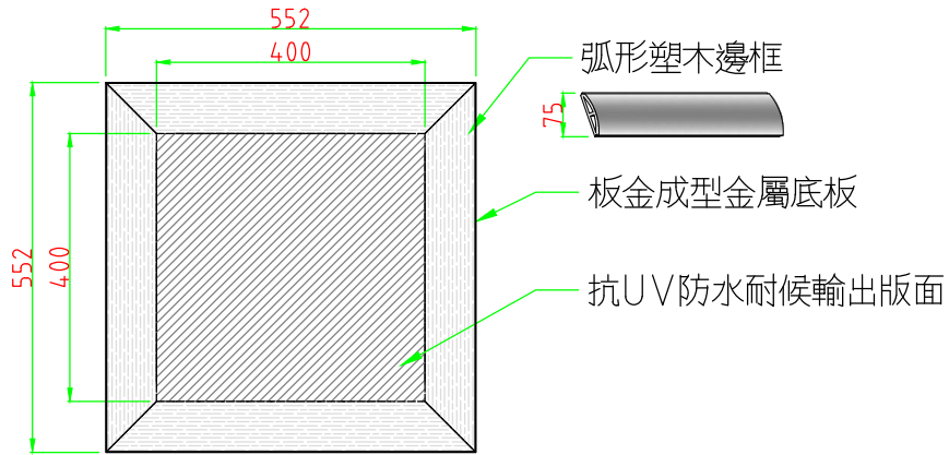
版面示意圖
