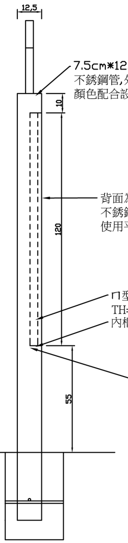
解說牌 側立面圖
