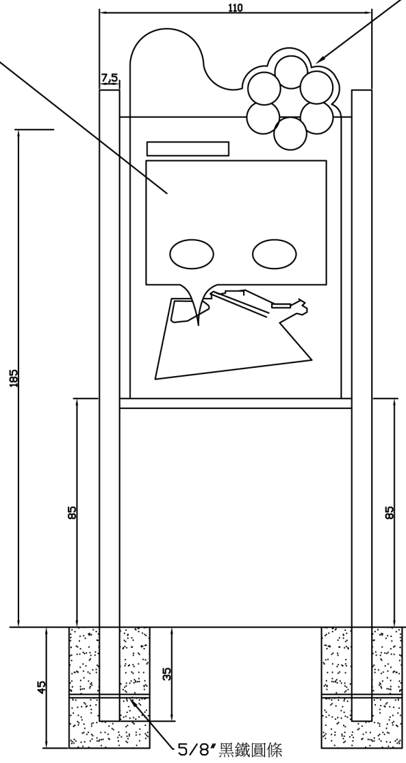
解說牌 正立面圖
